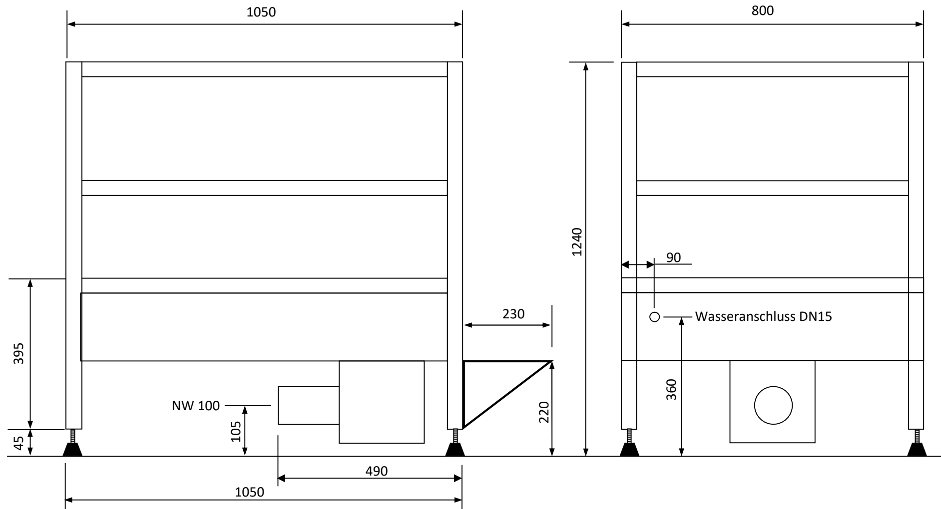
Stiefelwaschanlage STW 337-G Maßdetails
